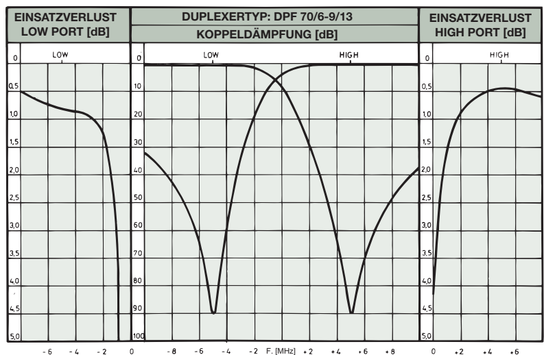
TYPISCHER KURVENVERLAUF @ 10 MHz ABSTAND
